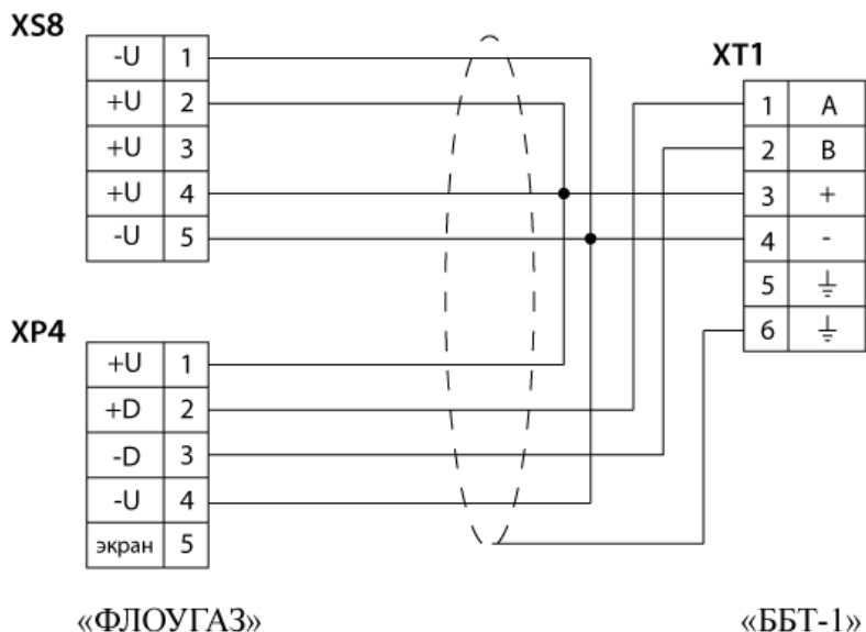
Рисунок 2. Схема подключения блока.
